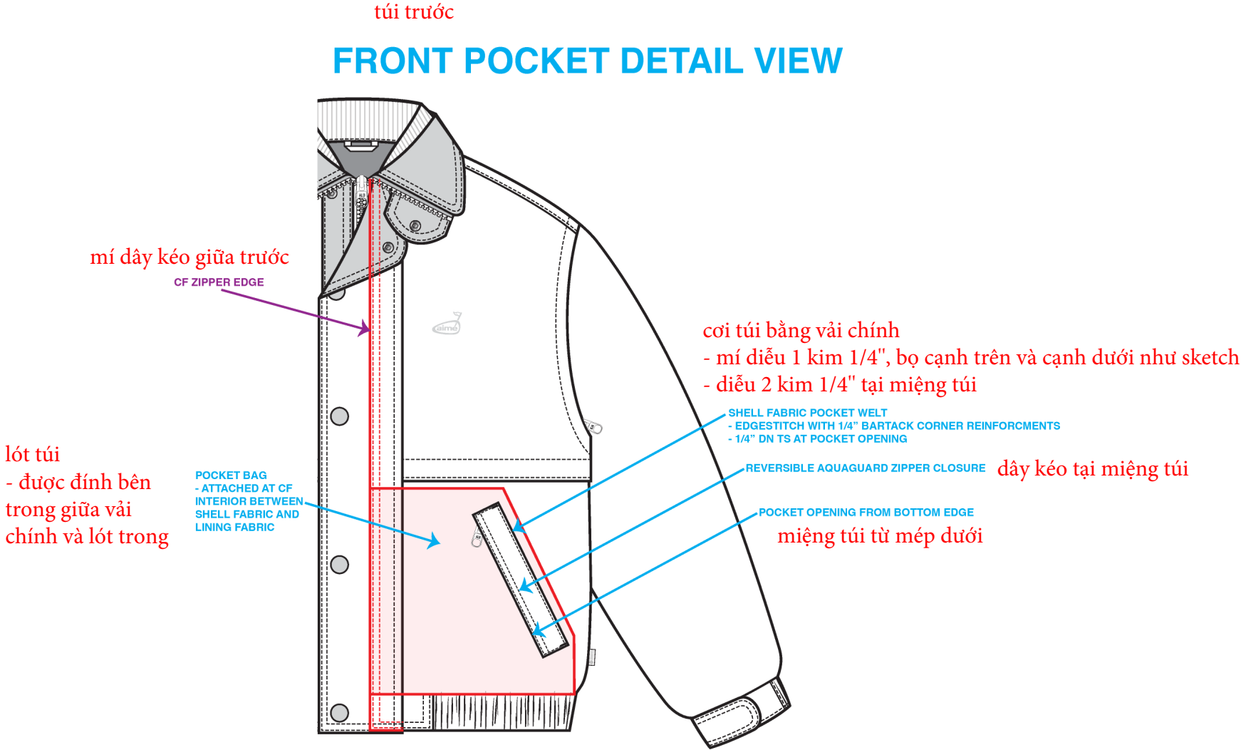
10_DETAIL-1
